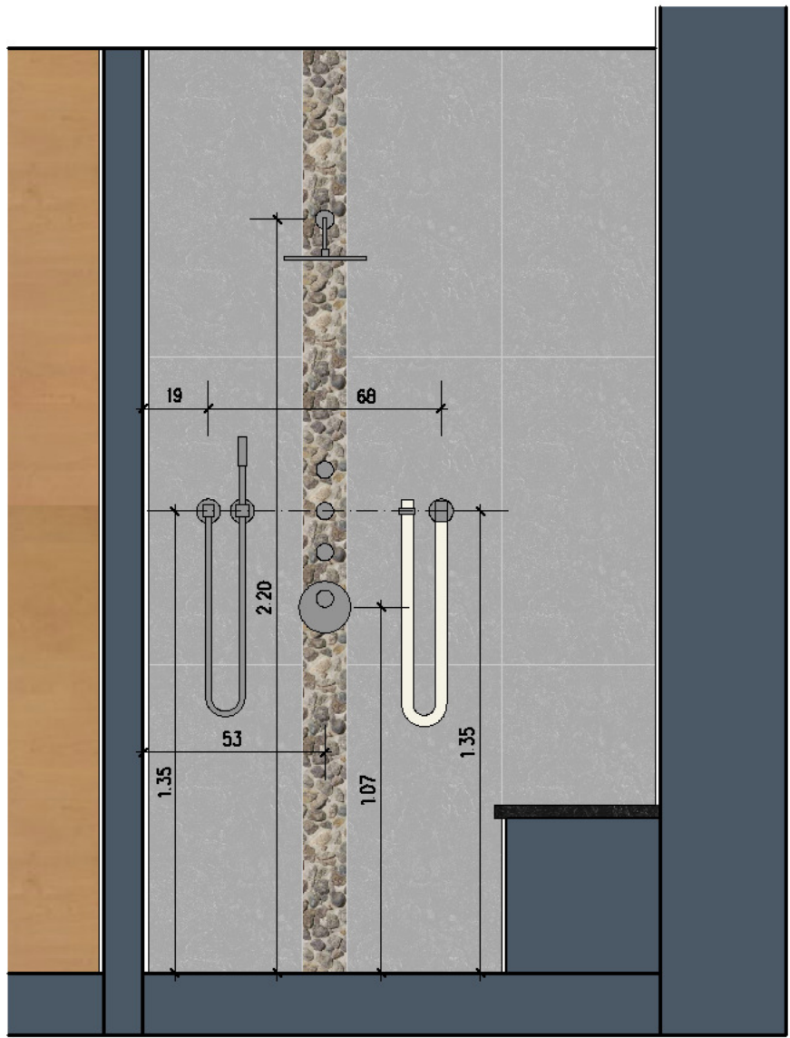
ANSICHT D
