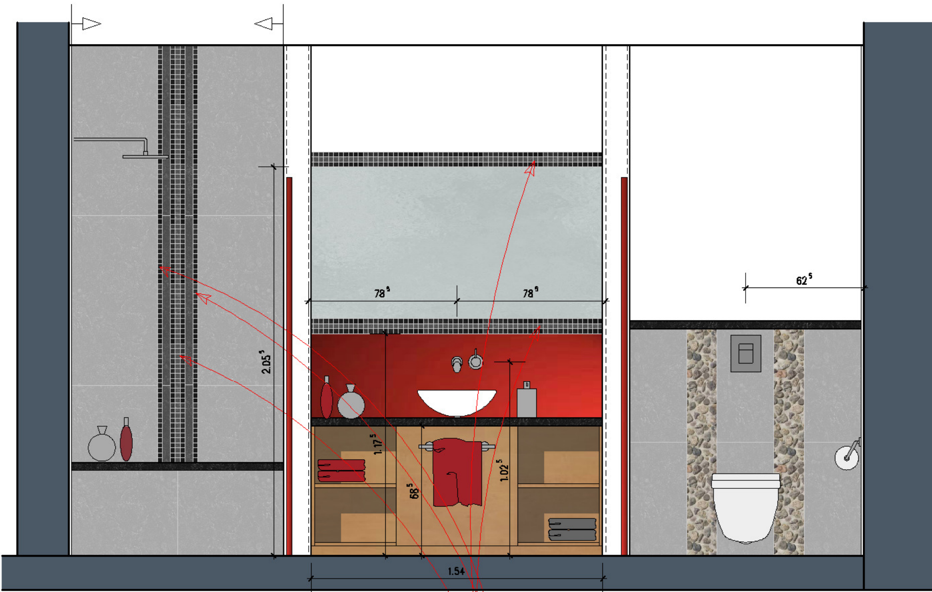
ANSICHT B
