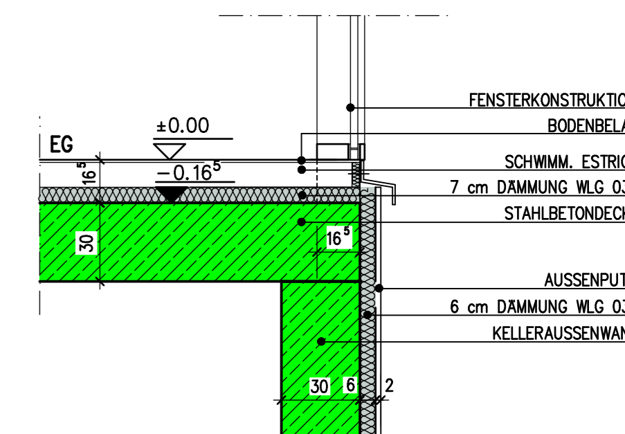
FASSADENSCHNITT 1 M. 1:20
