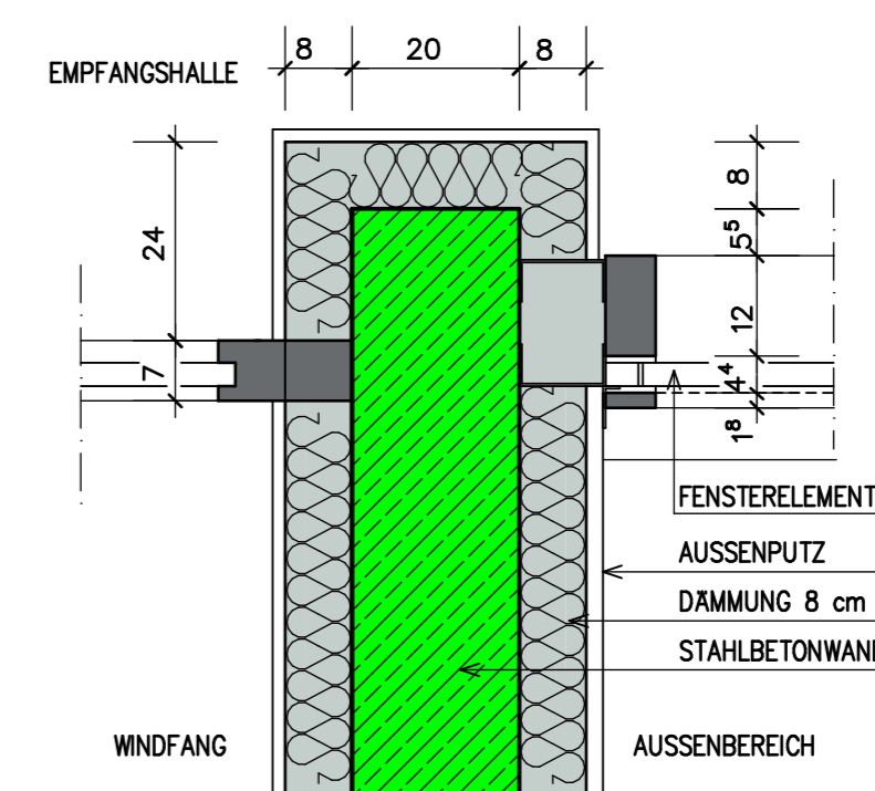
DETAIL EG2 M. 1:10
